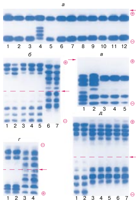
Рис. 2. Межвидовые и межродовые различия, обнаруживаемые при электрофоретическом исследовании множественных гемоглобинов рыб семейства лососевых ( Salmonidae ) (из [4]): а: 1–3 и 5–12 – кета, Oncorhynchus keta ; 4 – кижуч, O. kisutch (электрофорез в агаровом геле); б: 1–5 – голец, Salvelinus leucomaenis ; 6, 7 – горбуша, Oncorhynchus gorbusha (электрофорез в крахмальном геле); в: 1 – O. gorbusha ; 2 – гибрид F_1 ; 3–5 – сима, Oncorhynchus masu (электрофорез в агаровом геле); г: 1, 2 – O. keta ; 3, 4 – O. gorbusha ; д: 1, 2 – Salvelinus leucomaenis ; 3–7 – O. keta (электрофорез в крахмальном геле). Стрелка обозначает стартовую позицию, “+” и “–” – анод и катод соответственно. Хорошо видно, как при полном генотипическом тождестве особей внутри вида наблюдаются качественные межвидовые различия. Более детальную информацию о методе электрофоретического разделения генетически контролируемых вариантов белков см. в статье Ю.П. Алтухова “Генетика популяций и сохранение биоразнообразия” (СОЖ. 1995. № 1)
